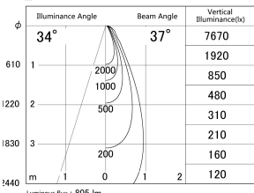
Luminous flux : 805 lm
