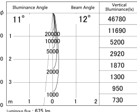
■ Direct Horizontal Illuminance DD155-0810MW9035
