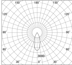
Luminous flux : 1215 lm
