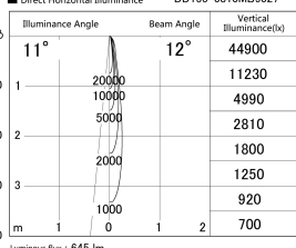
■ Direct Horizontal Illuminance DD155-0810MB9027
