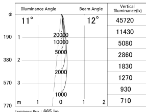
■ Direct Horizontal Illuminance DD155-0810DW9035
