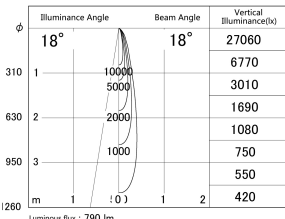
■ Direct Horizontal Illuminance DD155-0815DW9040
