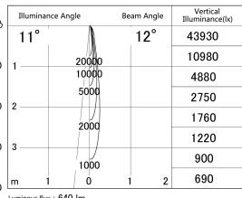
■ Direct Horizontal Illuminance DD155-0810DB9027
