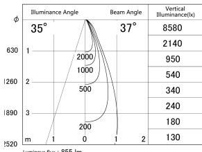
■ Direct Horizontal Illuminance DD155-0835WW9040
