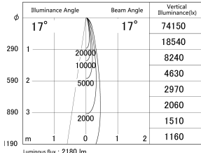
■ Direct Horizontal Illuminance DD155-2015WW9040
