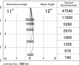
■ Direct Horizontal Illuminance DD155-0810MW9040-FX
