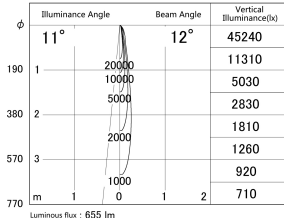
■ Direct Horizontal Illuminance DD155-0810DW9030-FX
